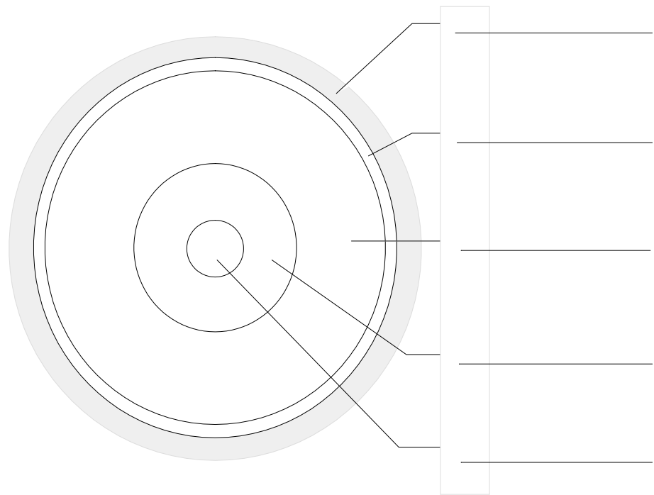
Structure interne de la Terre
